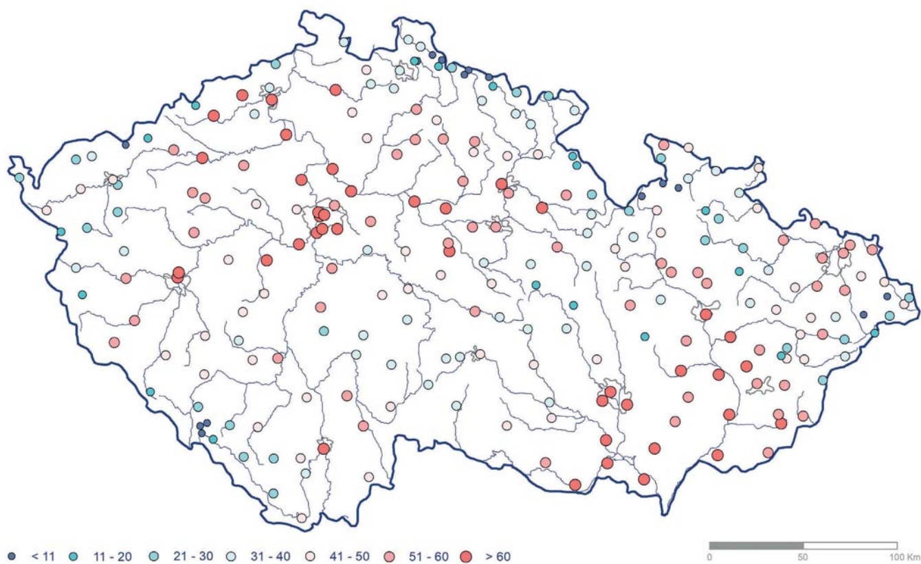
Obr. 2.16 Počet letních dní (denní maximum teploty vzduchu \geq 25 °C) v roce 2020.
