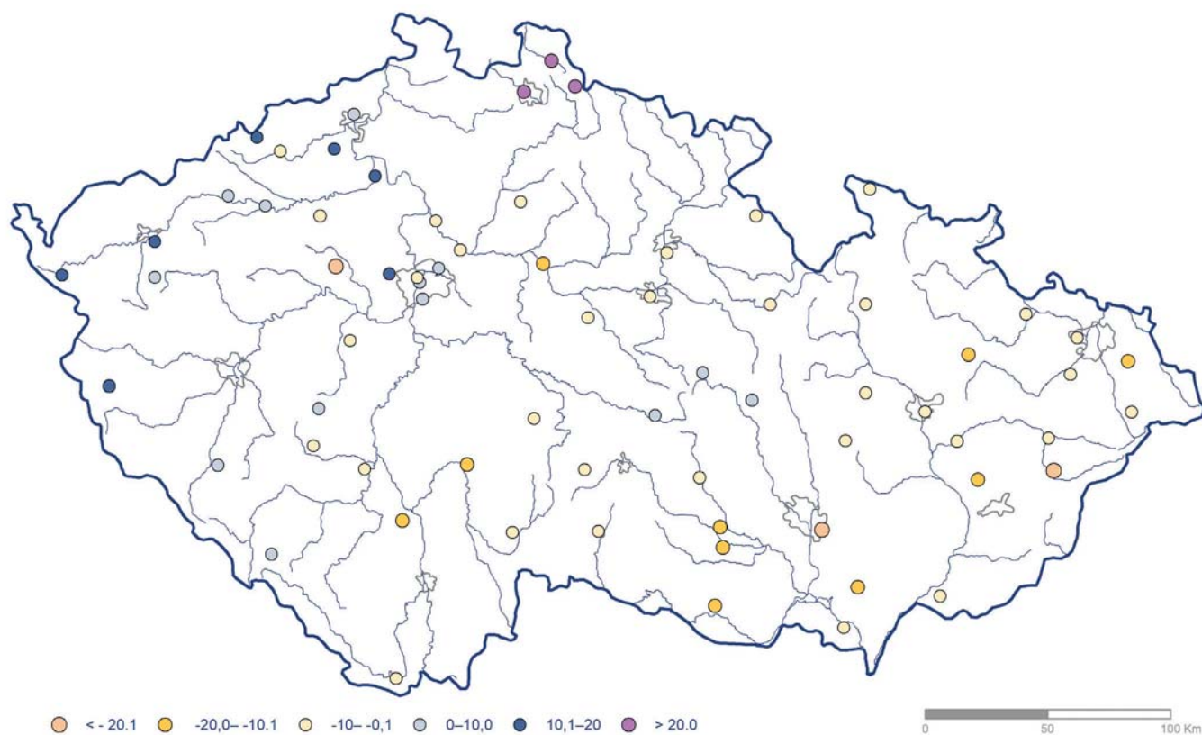
Obr. 5.6 Odchylna počtu zamračených dní v roce 2021 od normálu 1991–2020.
