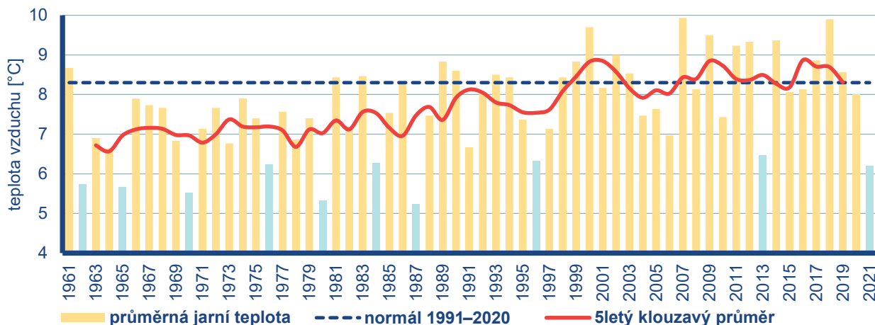
Obr. 7.3 Průměrná jarní teplota vzduchu na území ČR v letech 1961–2021. Modře jsou označeny hodnoty nižší než 6,5^{\circ}\text{C} .
