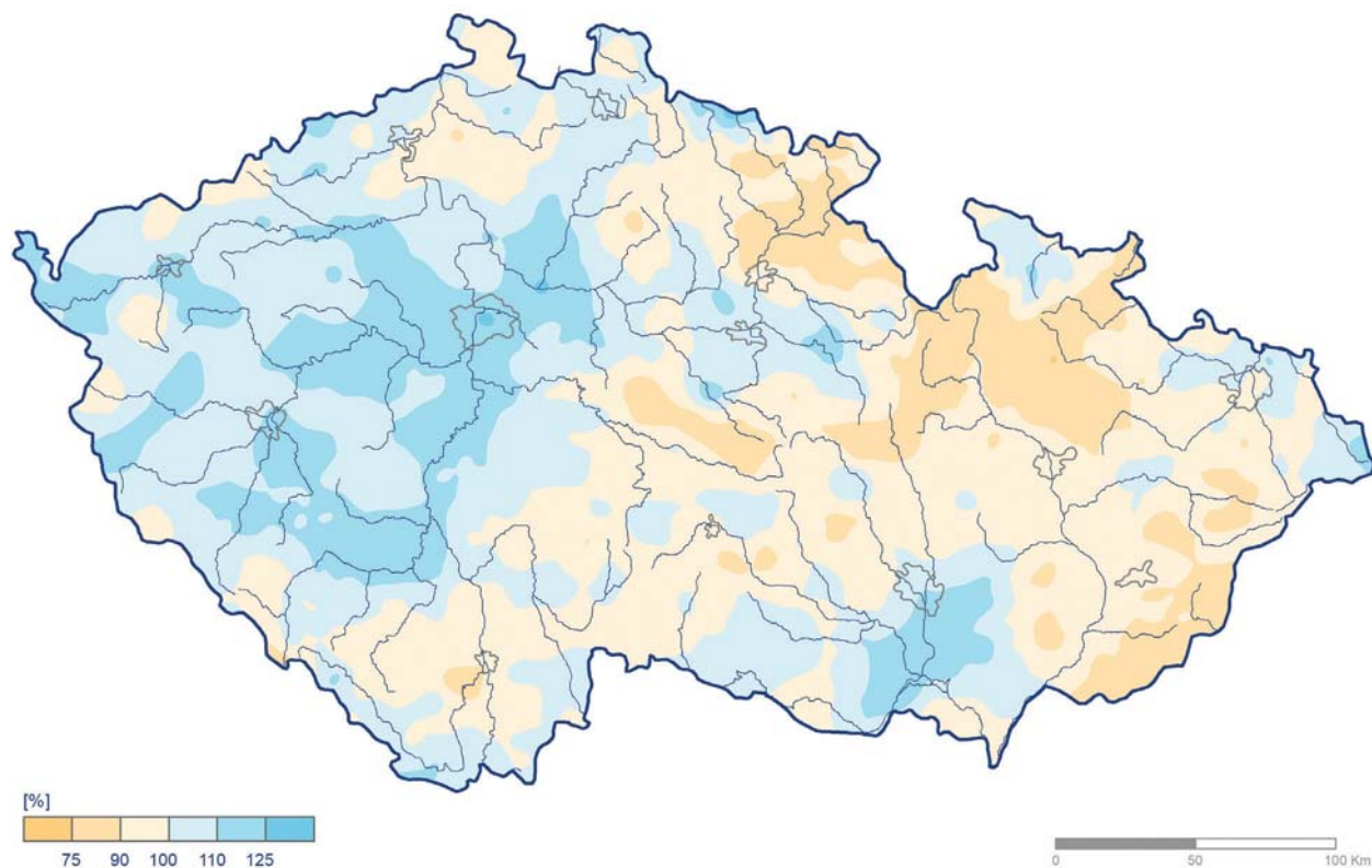
Obr. 3.2 Úhrn srážek v roce 2021 v % normálu 1991–2020.
