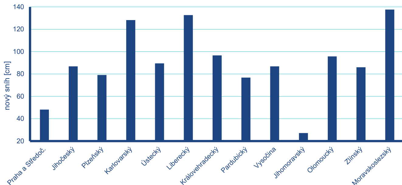
Obr. 4.3 Úhrn nového sněhu [cm] v sezoně 2020/2021 podle krajů.
