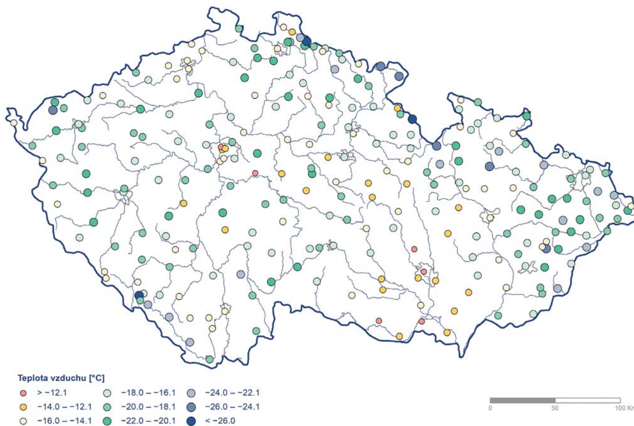
Obr. 2.12 Minimální teplota vzduchu [°C] v roce 2021.
