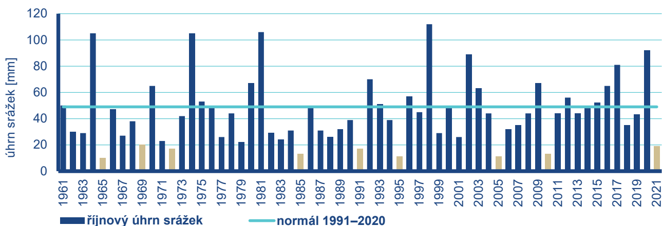
Obr. 7.7 Průměrný úhrn srážek za měsíc říjen na území ČR v letech 1961–2021. Okrově jsou vyznačeny hodnoty 20 mm a nižší.
