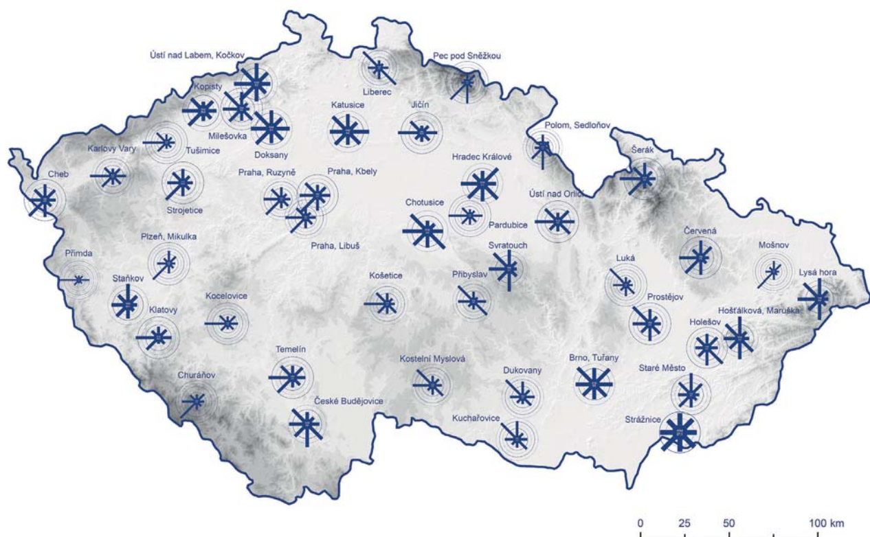
Obr. 6.4 Směr větru (větrná růžice) v roce 2021.
