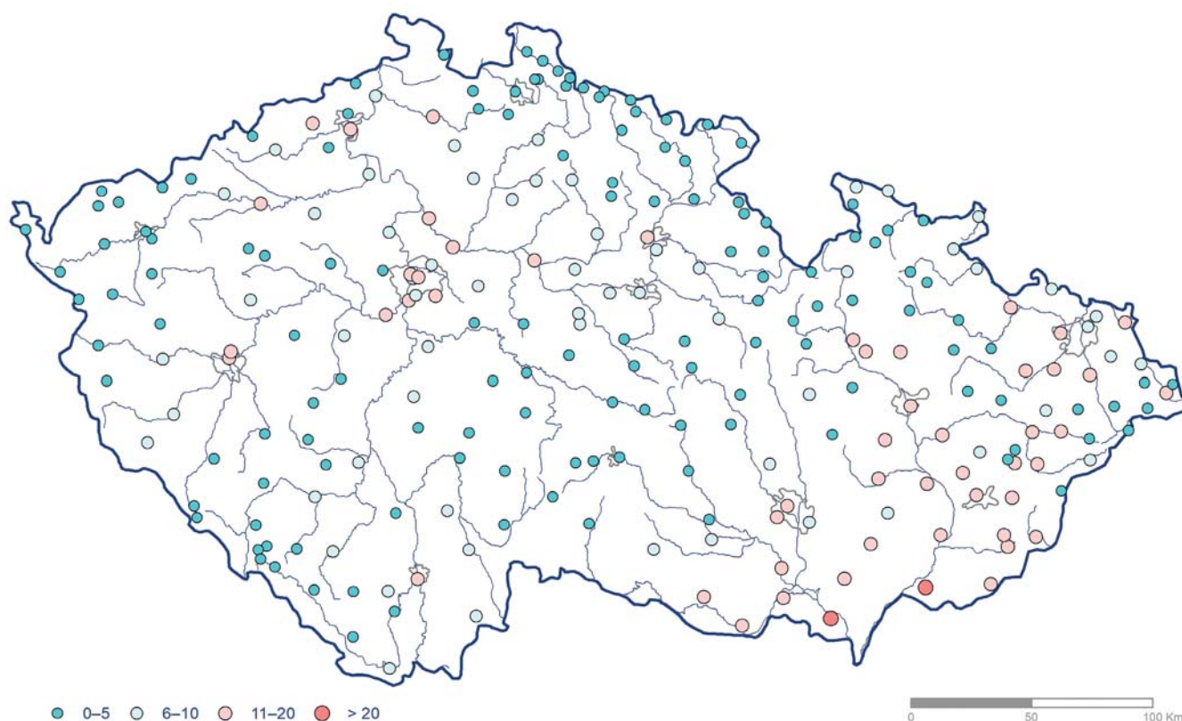
Obr. 2.19 Počet tropických dní (denní maximum teploty vzduchu \geq 30\text{ °C} ) v roce 2021.
