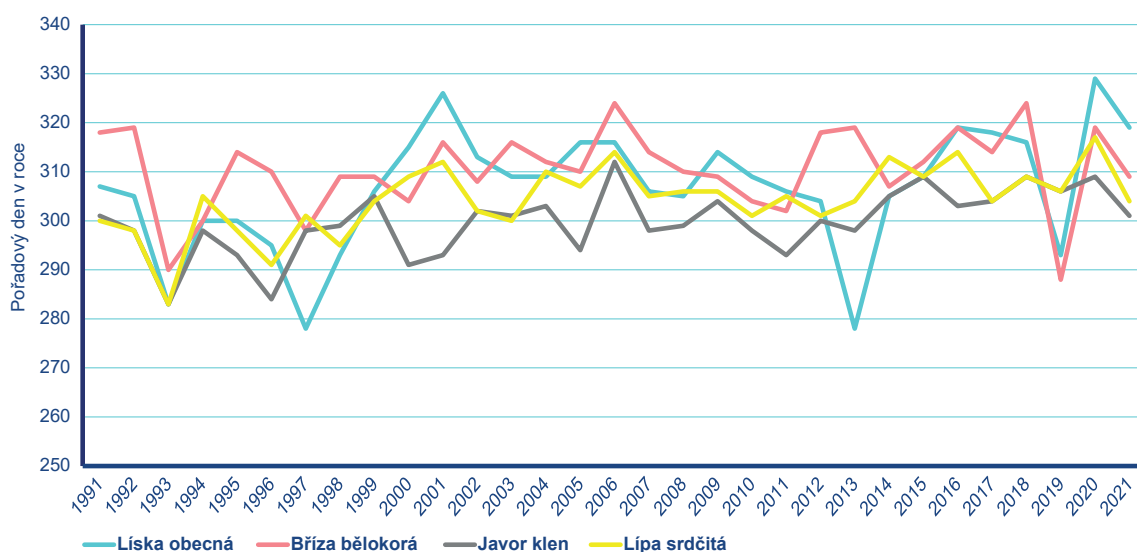
Obr. 8.4c Časový průběh fenologické fáze konec opadu listů za období 1991–2021 na stanici Chříbská.
