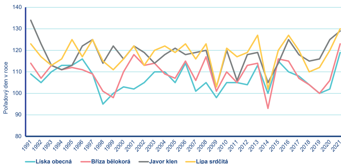
Obr. 8.4b Časový průběh fenologické fáze první listy za období 1991–2021 na stanici Chříbská.
