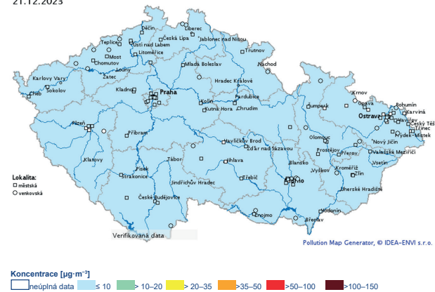
24hodinová průměrná koncentrace částic PM 10 , 21. 12. 2023.
