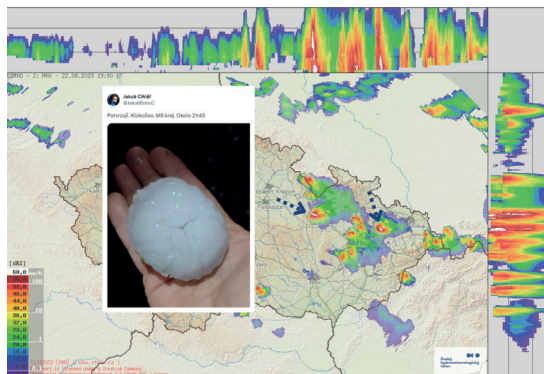
Radarový snímek ze dne 22. 8. 2023, kdy se vyskytly kroupy, které dosahovaly průměru až 8 cm.
