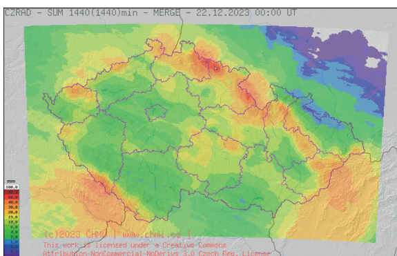
Denní srážkový úhrn 21. 12. 2023 na našem území.
