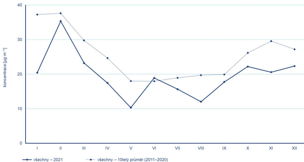
Obr. 13 Roční chod průměrných měsíčních koncentrací PM_{10} (průměry pro všechny stanice AIM), 2021
