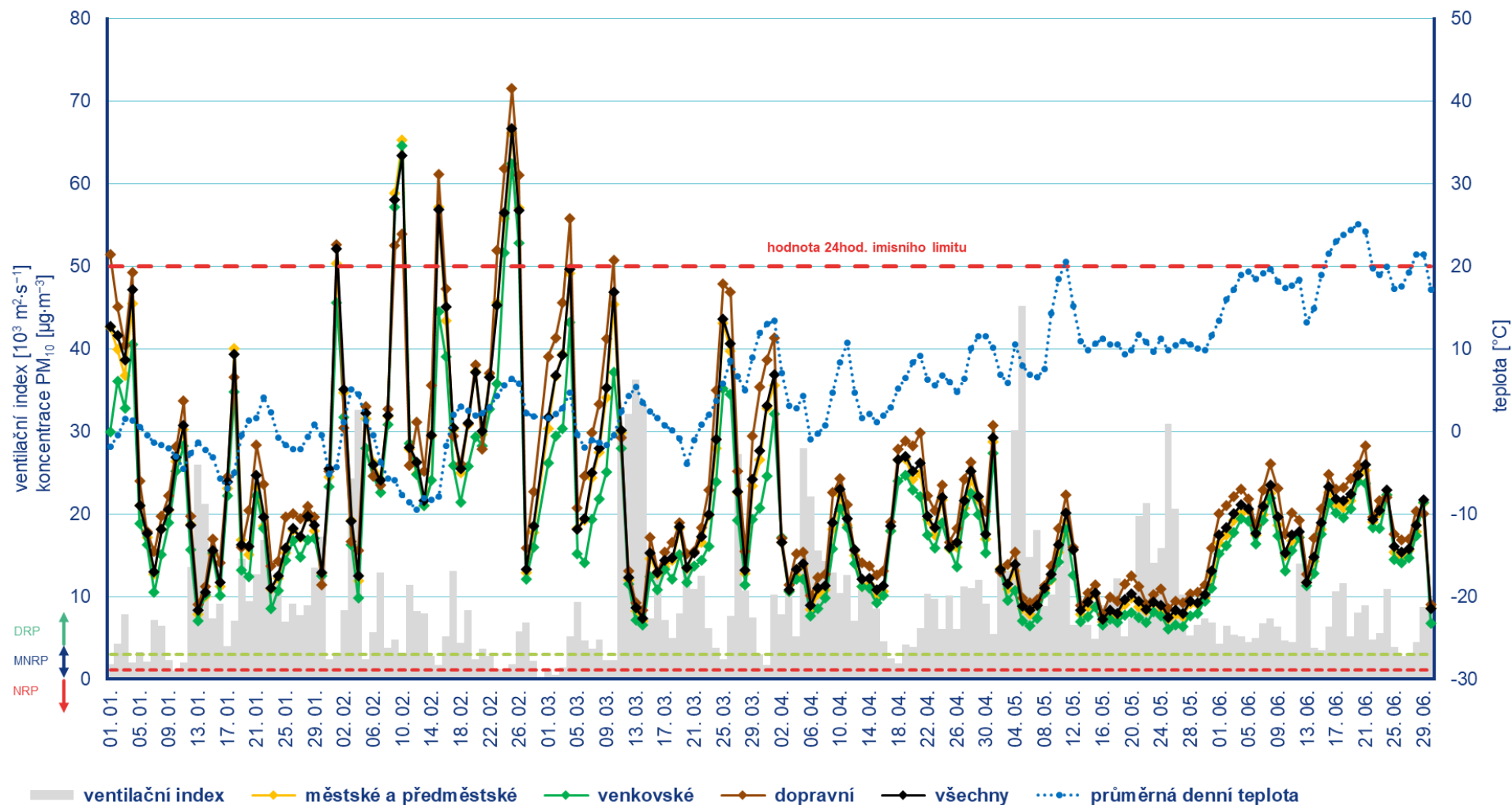
Obr. 28 Vývoj průměrných 24h koncentrací PM_{10} na stanicích AIM pro daný typ stanic a celorepublikového průměru teploty a ventilačního indexu (model ALADIN), leden–červen 2021
