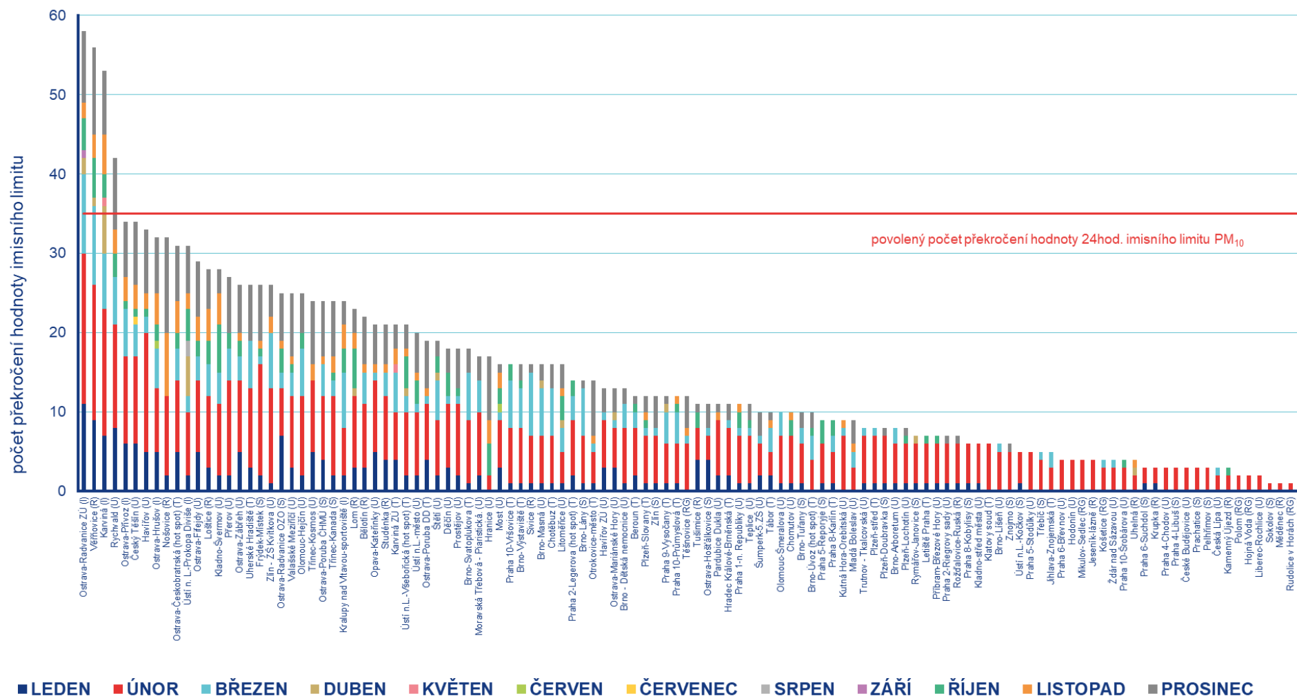
Obr. 10 Počet překročení hodnoty imisního limitu PM 10 (24h průměr) na měřicích stanicích AIM, 2021
