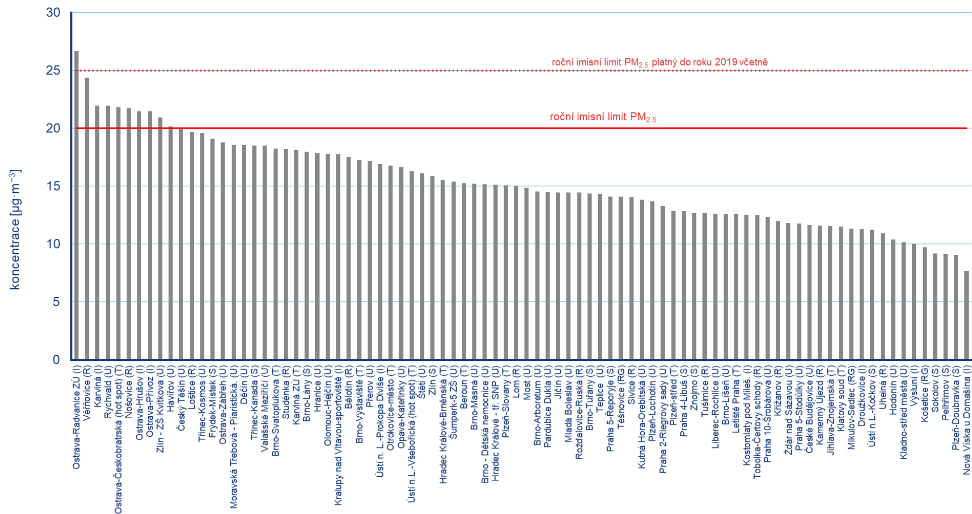
Obr. 15 Roční průměrná koncentrace \text{PM}_{2.5} na měřicích stanicích AIM, 2021
